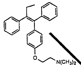
Tamoxifen
